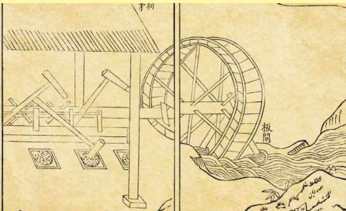
Martinet de broyage de minerai (水碓 shui dui); actionné par une roue à aubes (Tiangong Kaiwu, Song Yingxing 1637)
