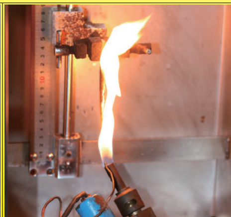
Eprouvette durant l'essai UL94 VO
