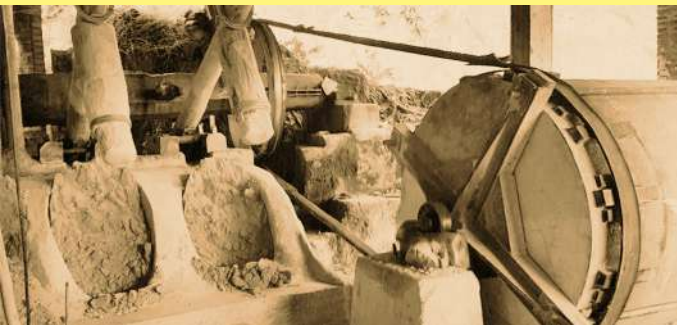
Machines de production traditionnelle des poudres (水碓 shui dui), utilisées pour fabriquer de la porcelaine électrique (collection privée)
