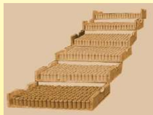
Séchage des porcelaines électriques après compactage au marteau (Collection privée)
